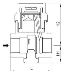
Type YSP-2
